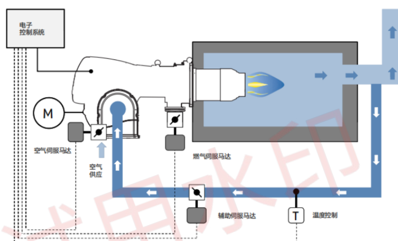
图 4-1 低氮燃烧器原理示意图
