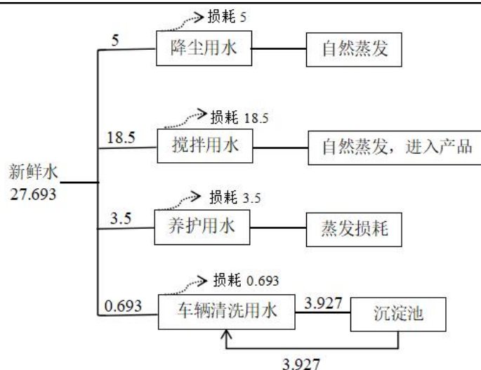
图 2-1 本项目水平衡图 (单位: m³/d)
