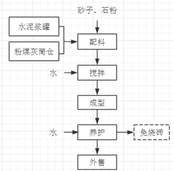
图 2-4 免烧砖生产线工艺及产污环节图
