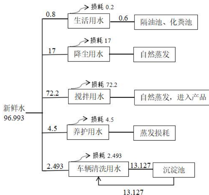
图 2-2 扩建后全厂水平衡图 (单位: m³/d)
